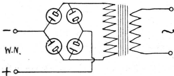
Rys. 7. — Ciekawa odmiana prostownika elektrolitycznego.
