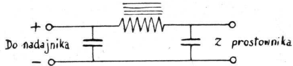
Rys. 5. — Schemat filtra.
