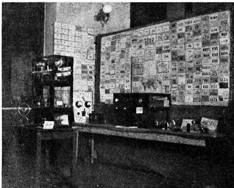
I-sza Ogólno-polska Wystawa Krótkofalowa we Lwowie. Stacja SP3AR, ze zbiorem kart pozaeuropejskich, odbiornikiem i tablicą rozdzielczą. Obok nadajniki SP3FV. Na pierwszym planie nadajnik SP3DM sterowany kryształem.
